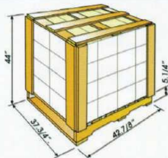
SA pallet Type A (44 Cartons)
